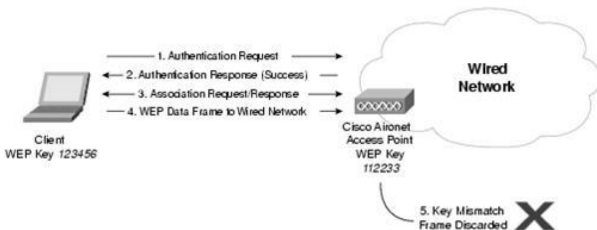
Fig: 2 Open Authentications
